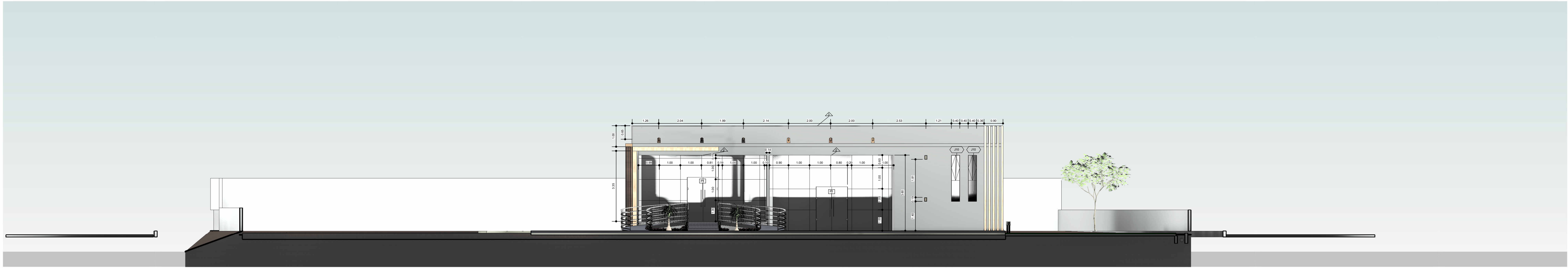
1 Corte AA 1 : 100
